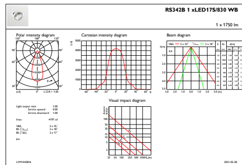
IFAS1_RS342B1xLED17S830WB
